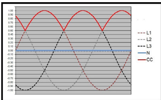
Figura 9 – Fem de salida de una fuente trifásica de media onda
